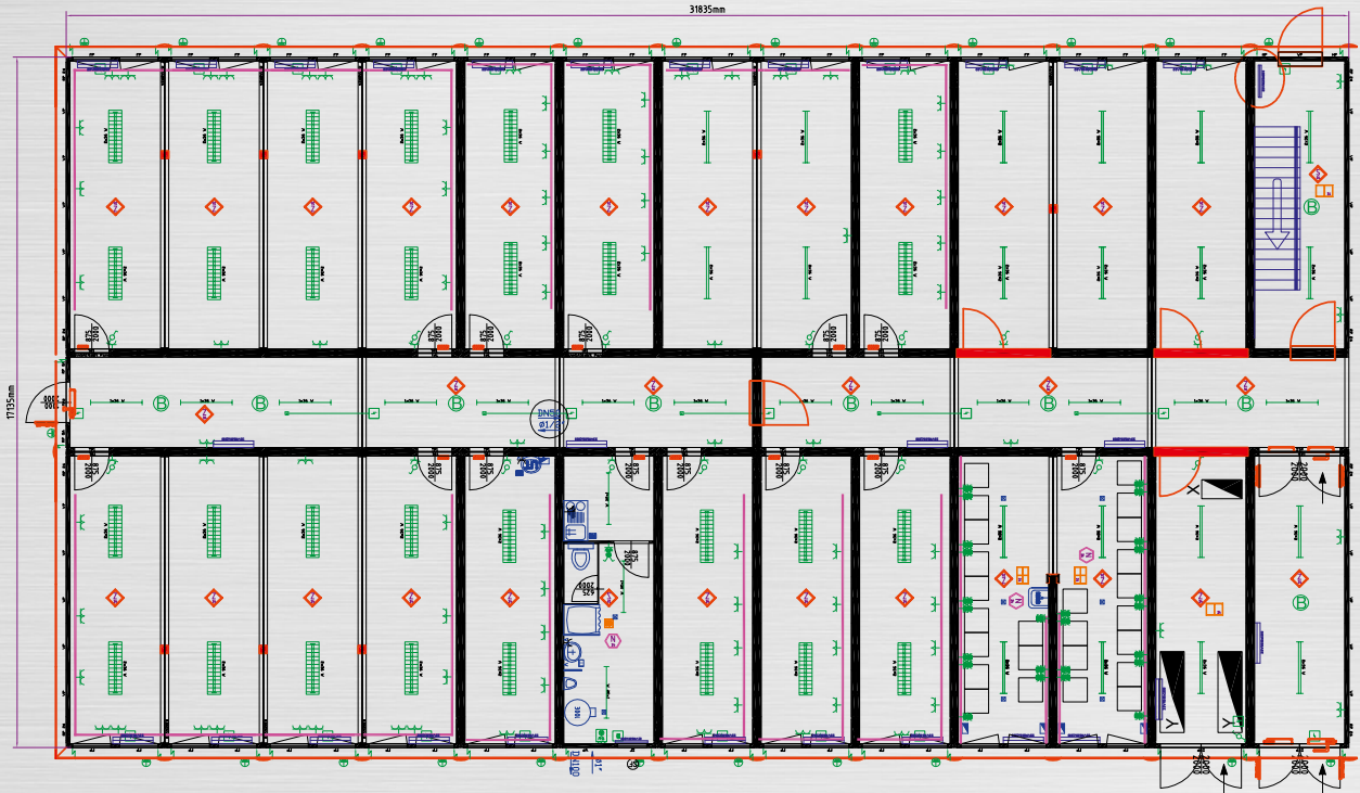
Planungsbeispiel Wohneinheit DE-Berlin für 150 Personen, 3-geschossige Anlage, Grundriss EG
