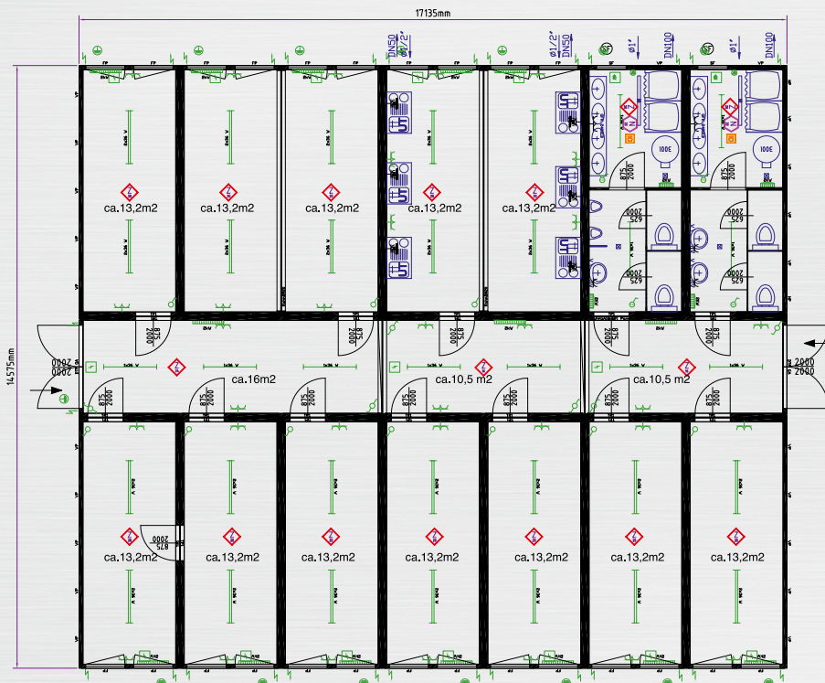
Planungsbeispiel Wohneinheit für 16 Personen – 3D Ansicht
