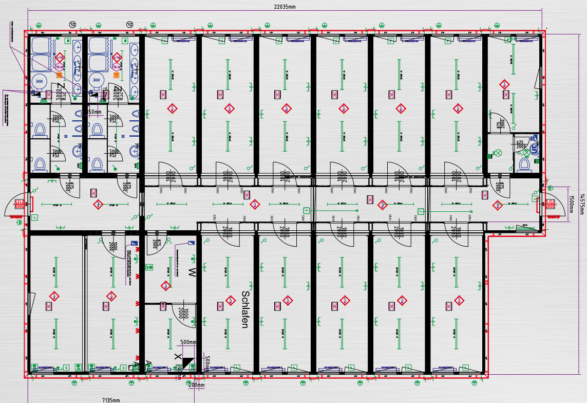
Planungsbeispiel Wohneinheit DE-Fellbach für 50 Personen, 2-geschossige Anlage, Grundriss EG
